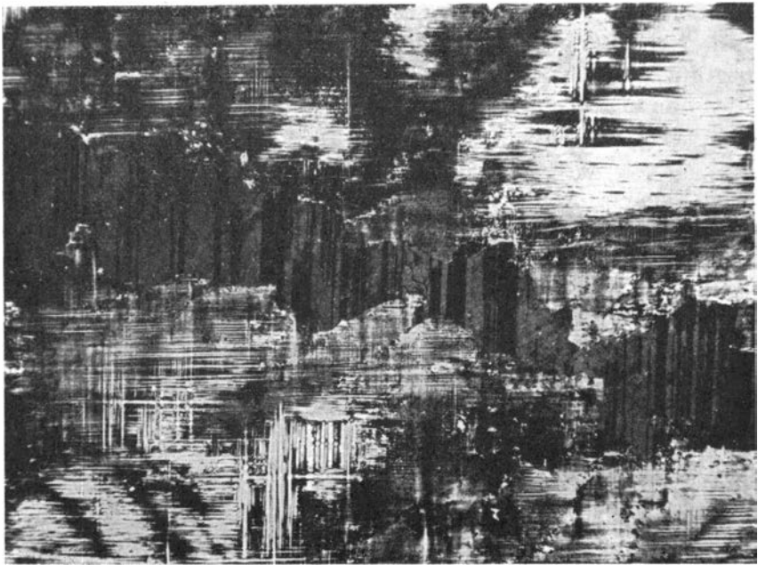
Figur 1. Dünnschliff parallel (001) von Mikrokl inperthit. Canada. (Näherer Fundort unbekannt). Dünne Lamellen nach Albit-, Periklin- und Mikrokl ingesetz. An einigen Stellen ist die Mikrokl ingitterung besonders fein ausgebildet. Man beachte auch die Gebiete mit einheitlicher Auslöschung (optisch »monoklin«) infolge submikroskopischer Verzwilligung. In der Mitte Makroalbit (»vein«-perthite) nach Albitgesetz verzwilligt. (Bildlänge = 2,5 mm, Nic. +).
