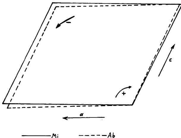
Figur 6. Gegenseitige Orientierung von Mikroklin (Mi) und perthitischem Albit (Ab) vom Typ I. b^*_{Mi} \parallel b^*_{Ab} . Schnitt (010) . \eta = [100]_{Mi} \wedge [100]_{Ab} \cdot \beta_{Mi} \simeq 116^\circ 00' \beta_{Ab} \simeq 116^\circ 40' .
